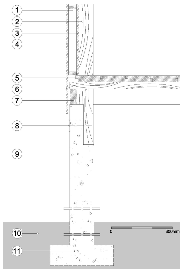
Pormenor tipo n.º 3
