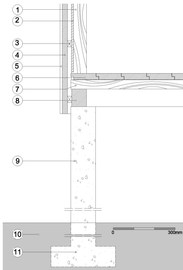
Pormenor tipo n.º 1
